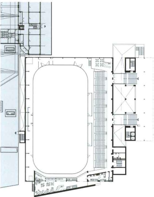
Půdorys přízemí — Ground floor plan
