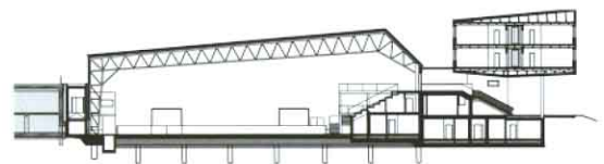
Řez — Section
